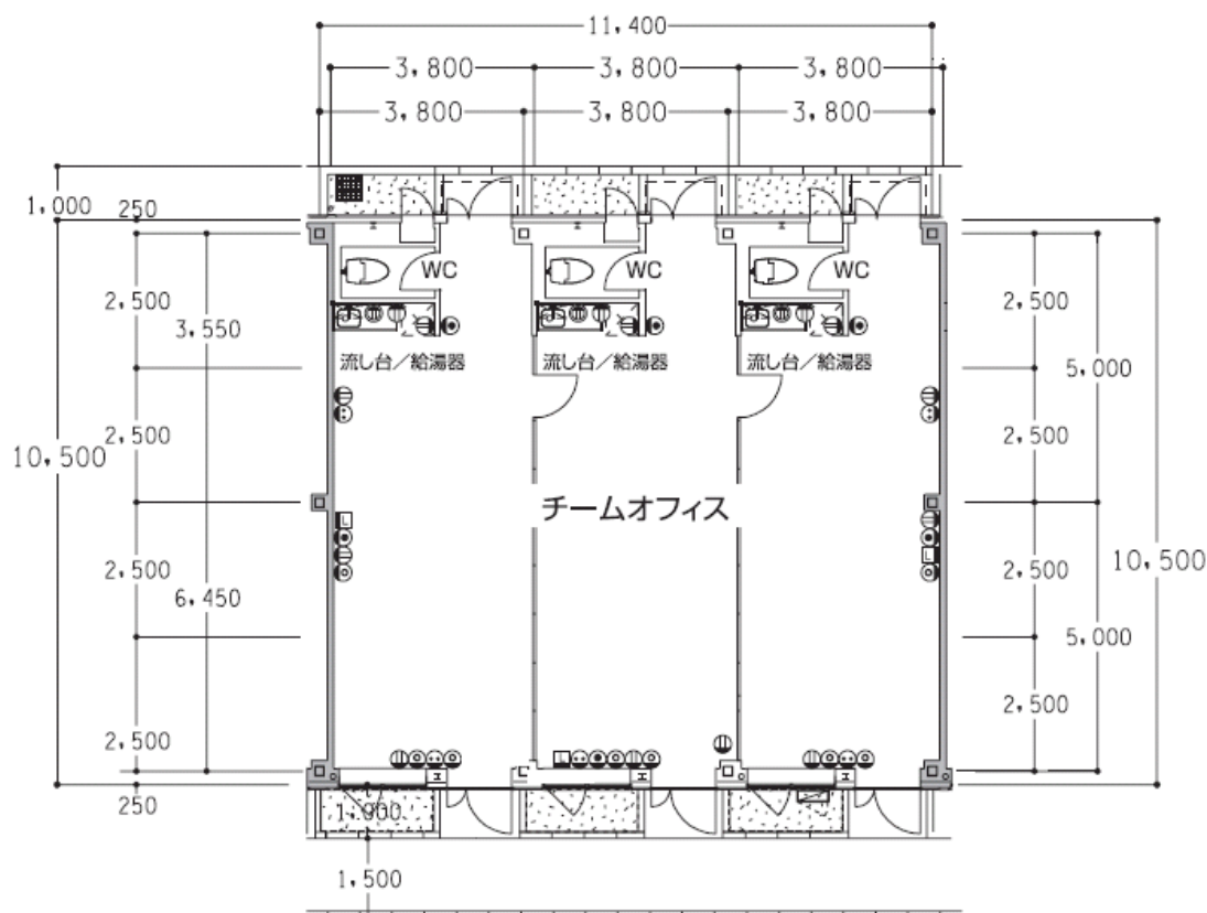
チームオフィス図面(B・C・D・E 棟)
