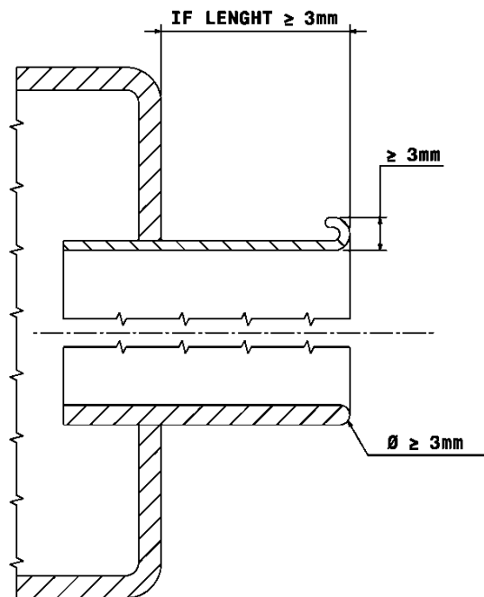
Figure 6 : Silencer edge
