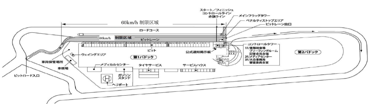
(b)ピット・パドック見取り図
